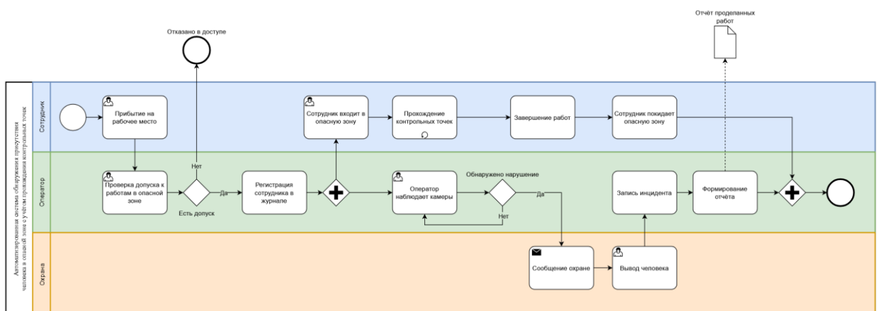
Рисунок 1. BPMN-диаграмма существующего бизнес-процесса
