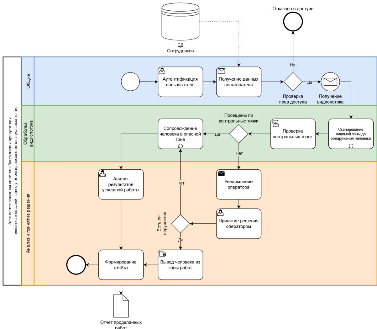
Рисунок 2. BPMN диаграмма бизнес-процесса обнаружения присутствия человека в опасной зоне
