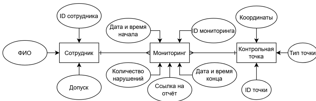
Рисунок 6. ER-диаграмма базы данных
