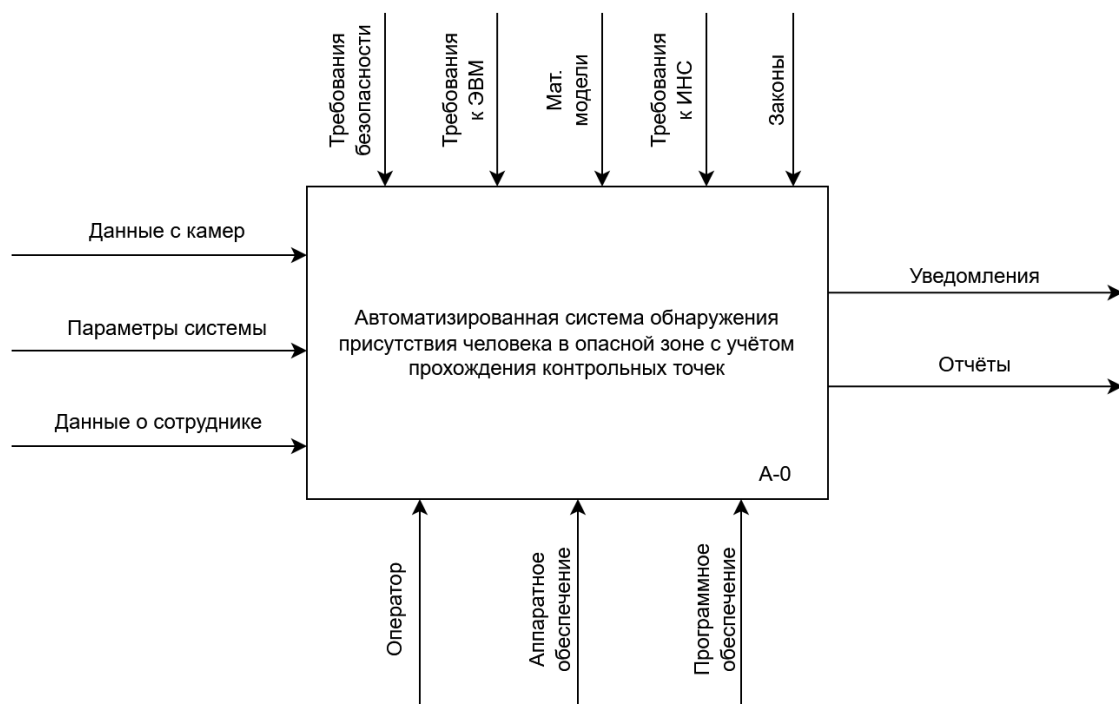
Рисунок 3. IDEF0 диаграмма системы
